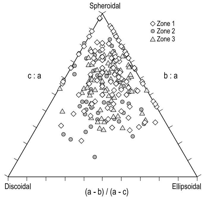
Figura 3. Diagrama de la esfericidad de los rodolitos de las zonas de muestreo 1, 2 y 3; cada punto es la esfericidad de un rodolito.
