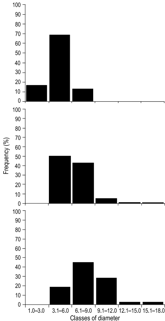
Figura 2. Frecuencia de distribución de las clases de diámetro de rodolitos (cm) por rango de profundidad: (a) zona 1, (b) zona 2, y (c) zona 3.
