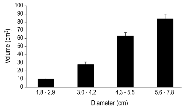
Figura 4. Volumen de los rodolitos en cuatro clases de diámetro de las zonas 1 y 2, que varían de 1.8 a 7.8 cm.
